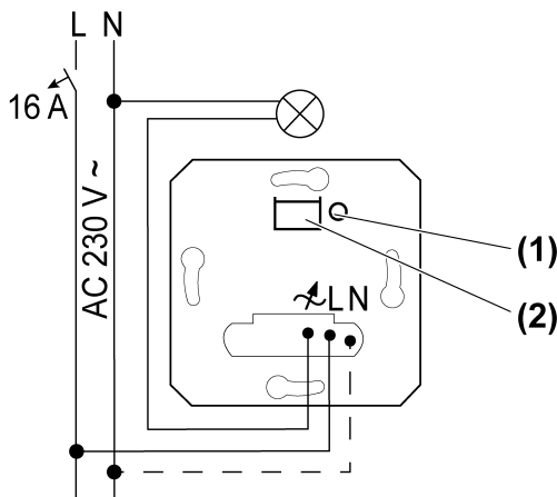
рисунок 1: Монтажная схема
